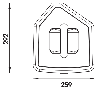
顶视
